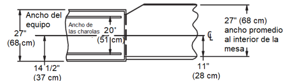
Disposición recomendada
