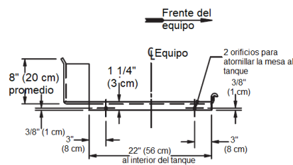
Vista mostrando las ubicaciones de los orificios en la parte trasera de la mesa
